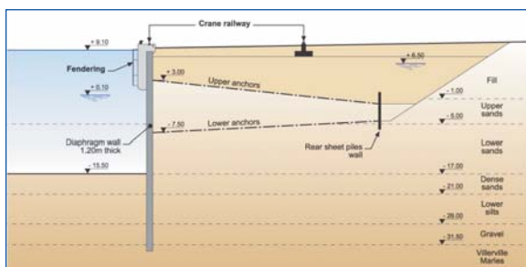
FRANCE - Le Havre Port 2000
